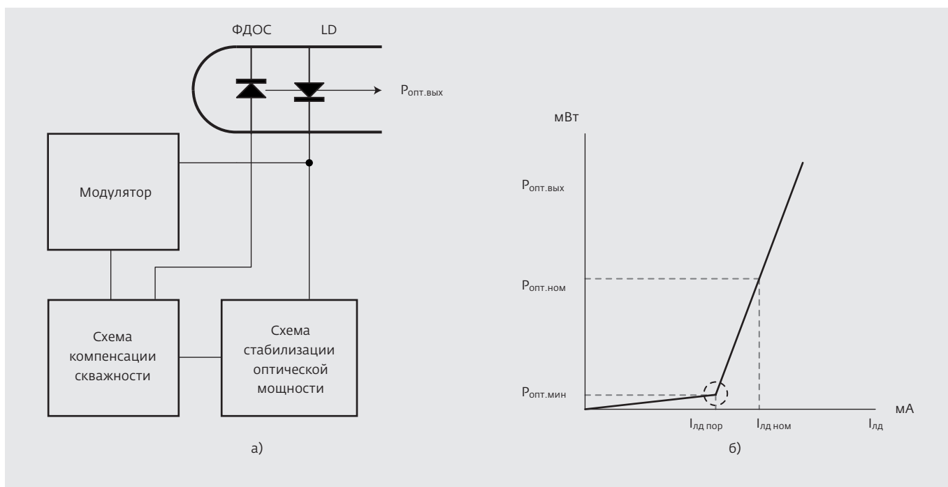
Рис.3. Функциональная схема оптического передающего устройства с компенсацией скважности входного сигнала (а) и выходная характеристика ЛД (б)
