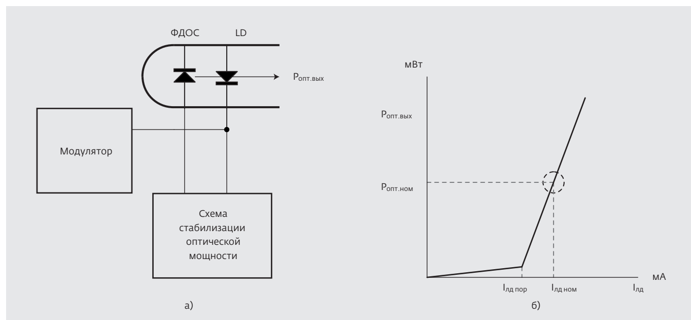
Рис.2. Функциональная схема оптического передающего устройства со стабилизацией среднего значения выходной оптической мощности (а) и выходная характеристика ЛД (б)
