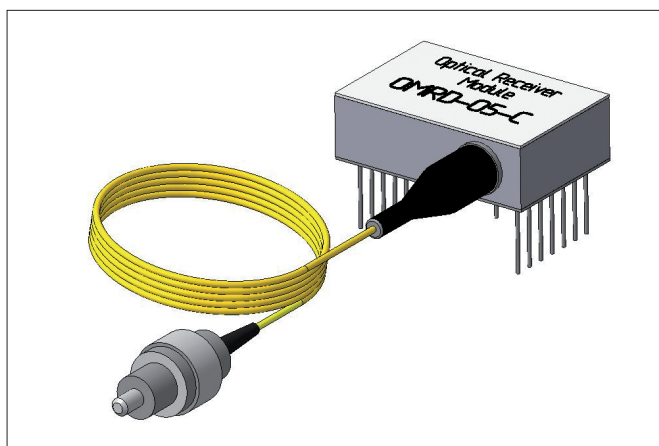
Рис.7. Волоконно-оптический приемный модуль OMRD-05-C
