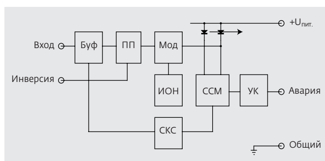
Рис.4. Функциональная схема волоконно-оптического передающего модуля ОМТД-05-С-с
