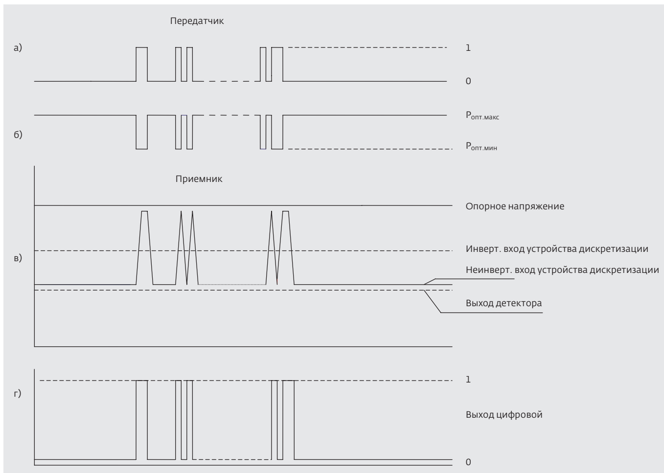
Рис.1. Эпюры входных и выходных электрических и оптических сигналов
