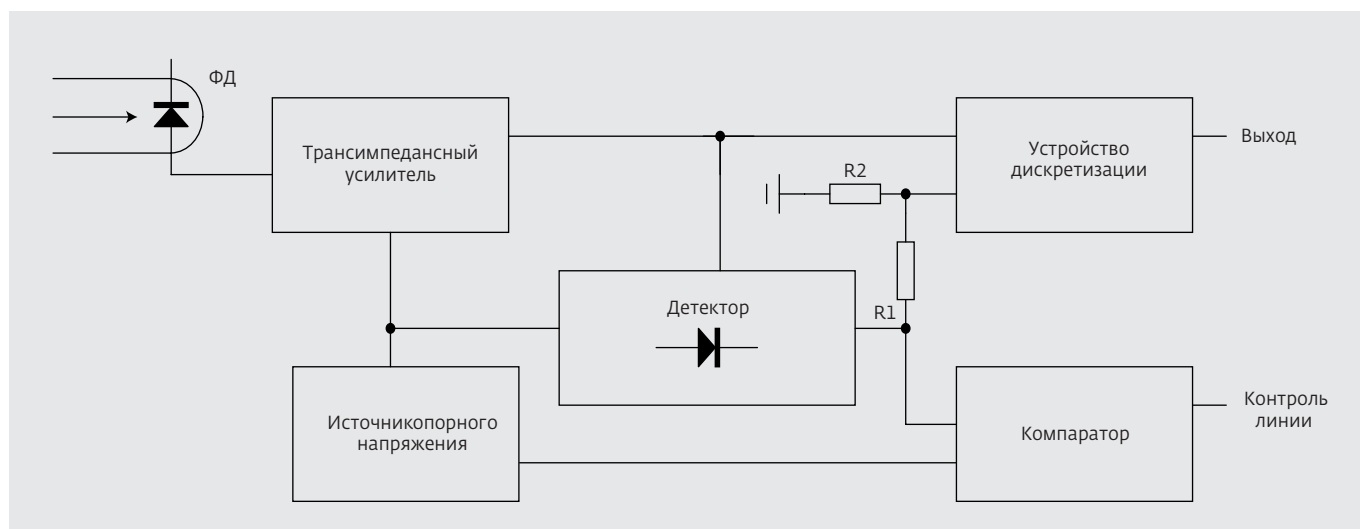
Рис.6. Функциональная схема волоконно-оптического приемника для приема одиночных оптических импульсов
